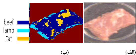
شکل ۳: الف) تصویر RGB ب) تحلیل به روش طبقه‌بندی SVM از گوشت گاو
